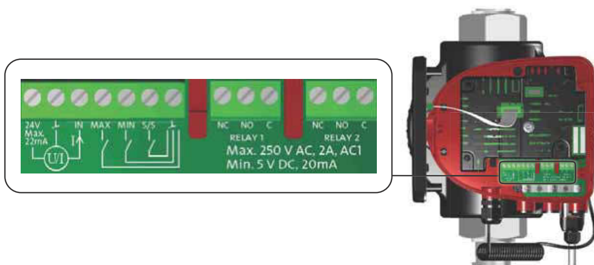
Rys. 51 Przykład połączeń w skrzynce sterowniczej dla wersji w wtyczkę
