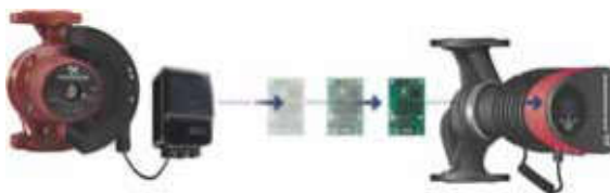
Rys. 66 Ponowne wykorzystanie modułu CIM
