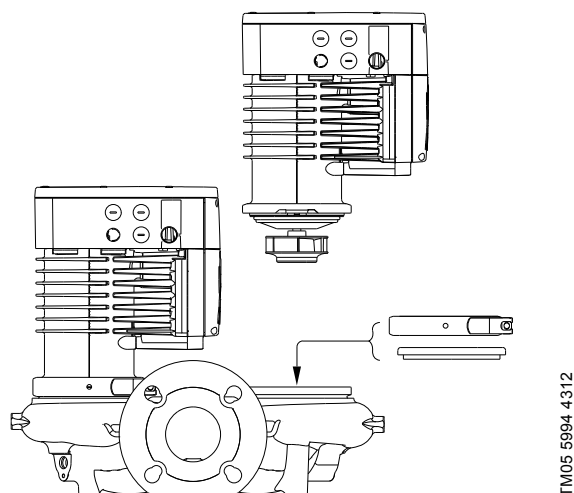
Rys. 70 Położenie kołnierza zaślepiającego
