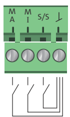
Rys. 54 Wejście cyfrowe w skrzynce sterowniczej
