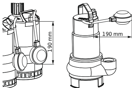
Fig. 5: Mocowanie i nastawianie wyłącznika pływakowego bez sterownika
