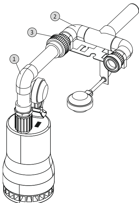
Fig. 13: Demontaż pompy
