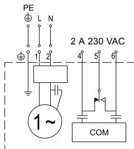
Obr. 3 Schéma zapojení jednofázových čerpadel
