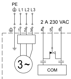
Obr. 4 Schéma zapojení trojfázových čerpadel
