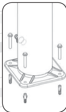
Obrázek 1 – Kotvení sprchy
