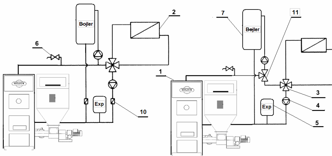
Schéma č. 6
