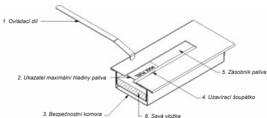
Obr. 2: Nádoba na biopálivo – průřez
