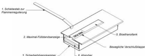
Zeichnung 2. Querschnitt der Sicherheitsbrennkammer
