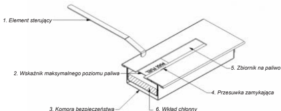
Rys. 2. Biopojemnik - przekrój
