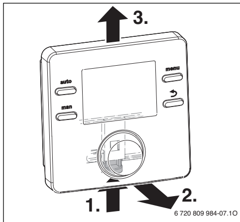
Obr. 10 Sejmutí regulace
