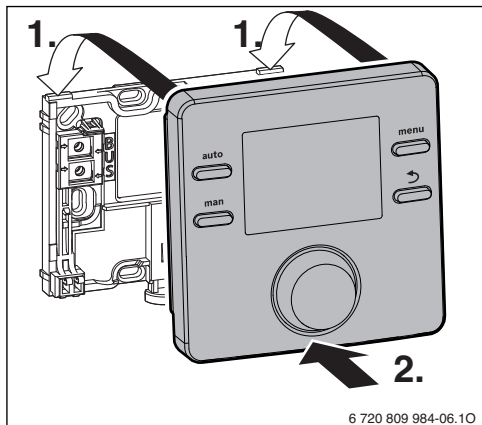
Obr. 9 Zavěšení regulace
