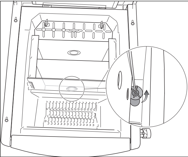
Obr. 24 Odstranění čistícího víka
