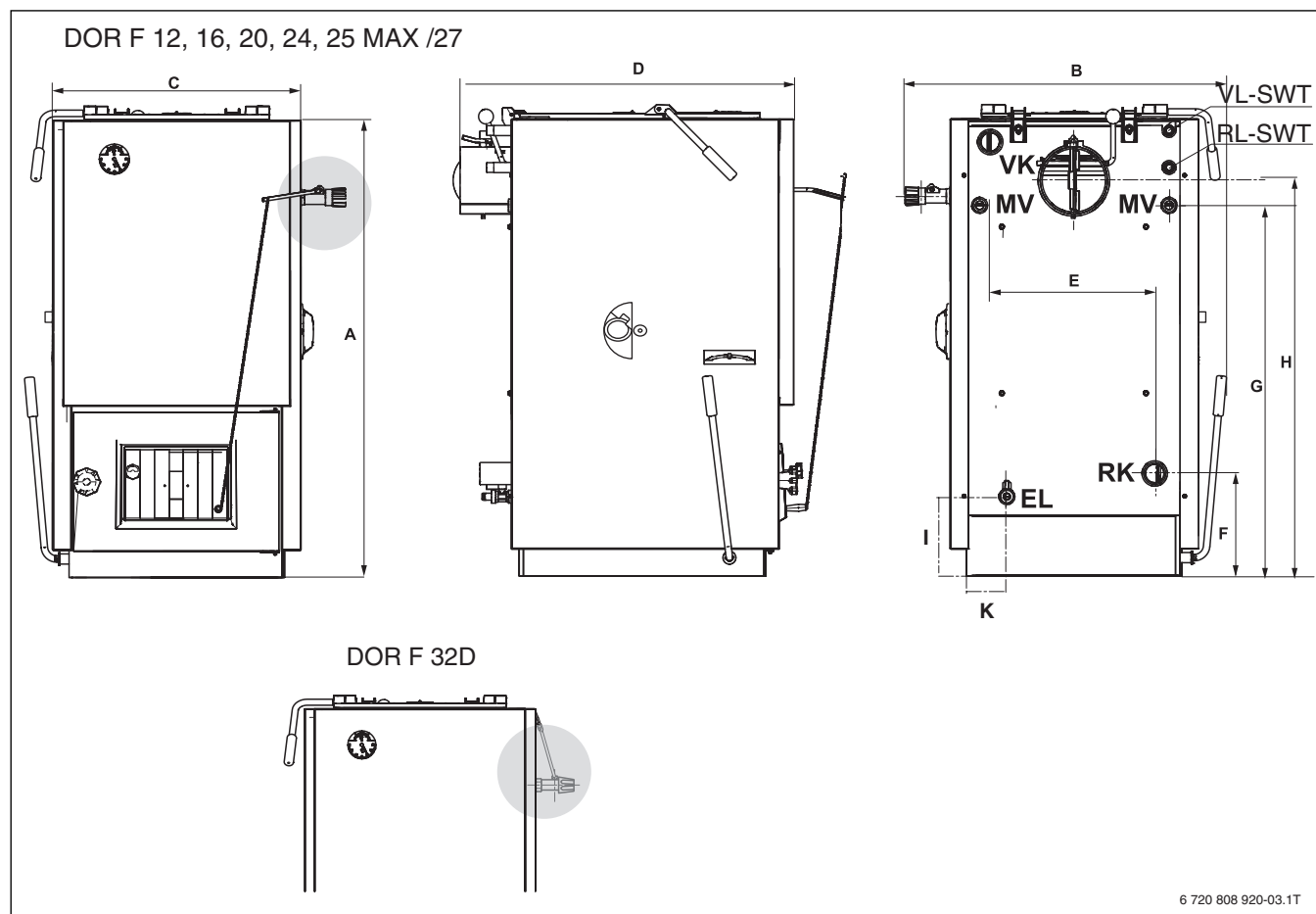
Obr. 5 Přípojky a rozměry
