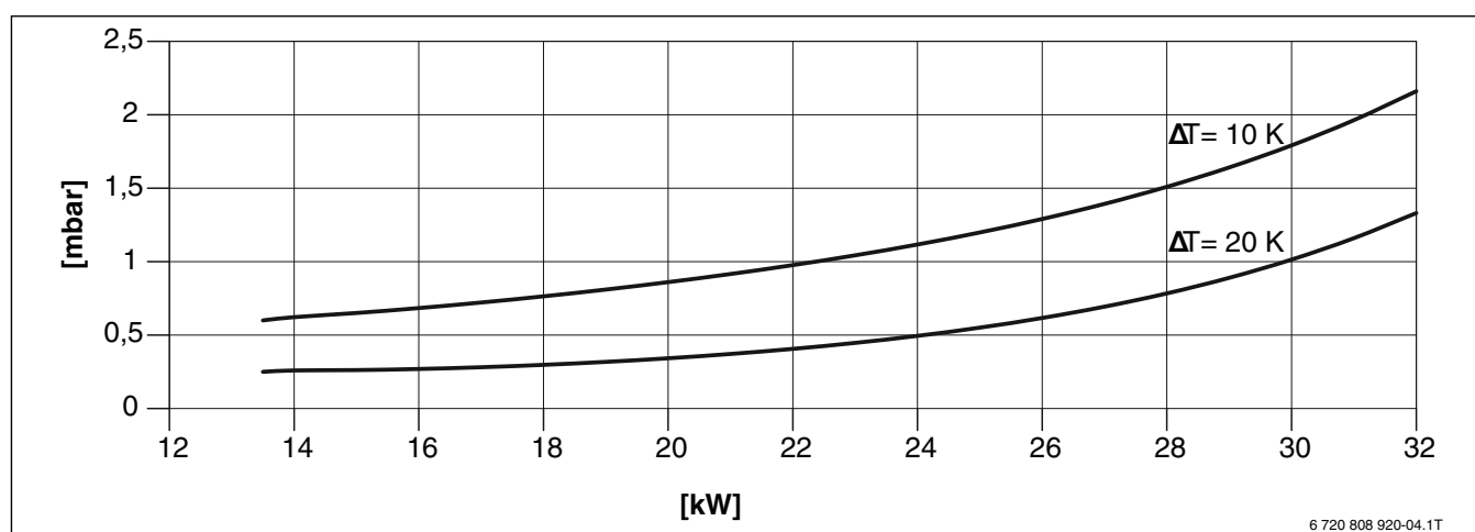
Obr. 6 Hydraulický odpor G 1½ "
