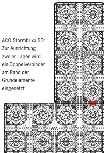
ACO Stormbrixx SD: Zwei zusammengesteckte Verbinder sichern die Ausrichtung der Pylonen zweier Einbaulagen
