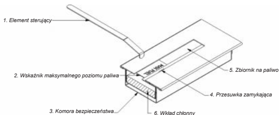
Rys. 2. Biopojemnik - przekrój
