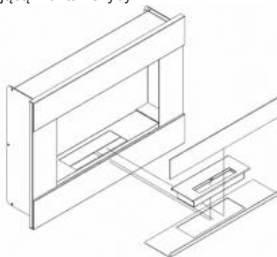
Rys. 3. Sposób montażu szyby w biokominkach Alpha, Bravo, Bravo 2, Charlie, Charlie2, Delta, Delta 2, Golf, Quat
