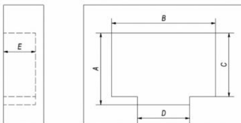
Obr. 10: Způsob dimenzování výklenku pro biokrbý
