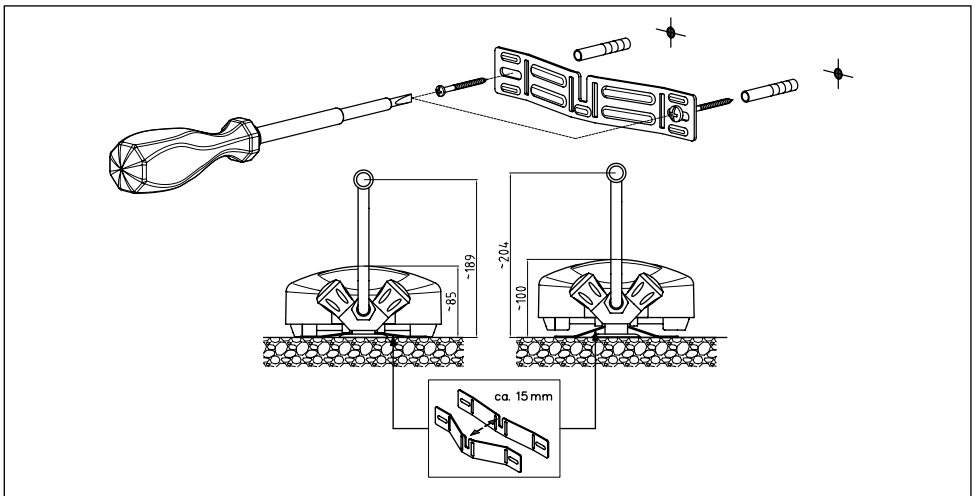
Afb. 5: "Montage van de metalen wandhouder" (maten in mm)
