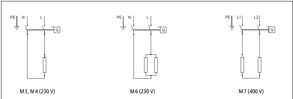
Abb. 8: »Schaltplan«
