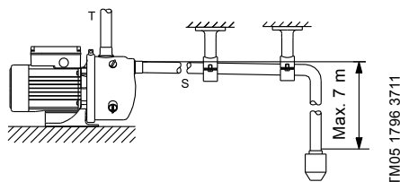
Fig. 2 Raccordement tuyauterie
