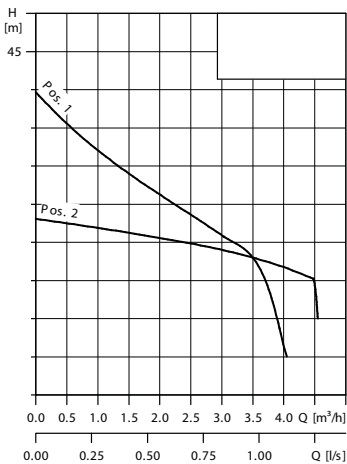
Рис. 3 Позиції кривої QH і клапану ежектора
