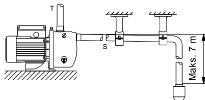
Rys. 2 Przyłącza rurowe
