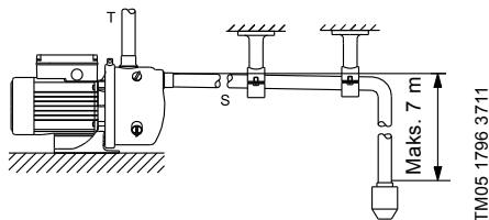
Joonis 2 Torude ühendamine
