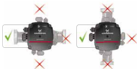
Abb. 6 Position des Schaltkastens, ALPHA SOLAR
