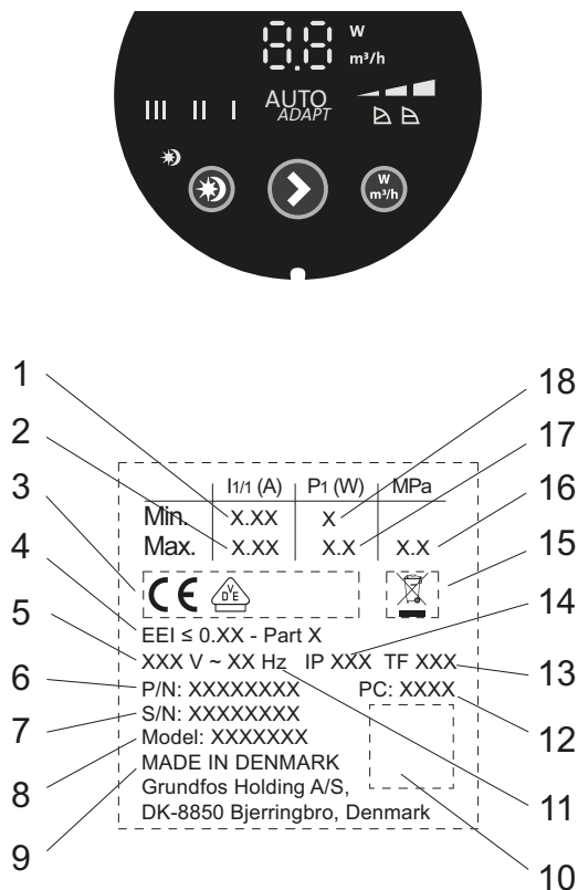
Abb. 18 Typenschild
