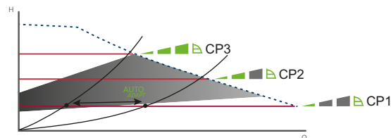
Abb. 24 Drei Konstantdruck-Kennlinien/-Einstellungen
