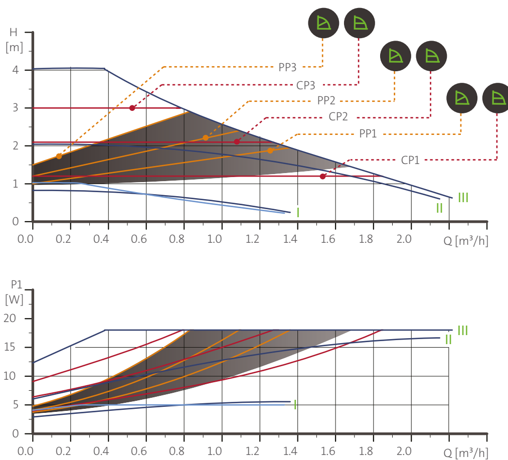
Abb. 40 ALPHA2 und ALPHA3, 25-40 A
