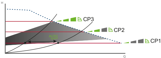
Abb. 26 Drei Konstantdruck-Kennlinien/-Einstellungen
