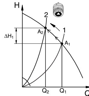
Abb. 11 Unregelmäßige Pumpe
