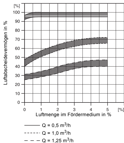
Abb. 20 Luftabscheidevermögen
