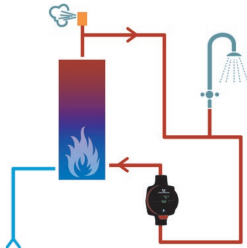
Abb. 6 Häusliches Warmwasserzirkulationssystem
