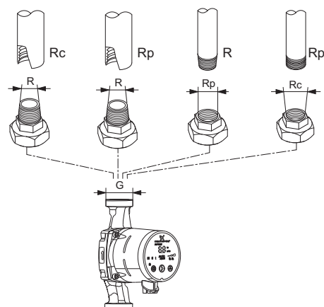
Abb. 25 Beispiele von Gewindearten und Kombinationsmöglichkeiten
