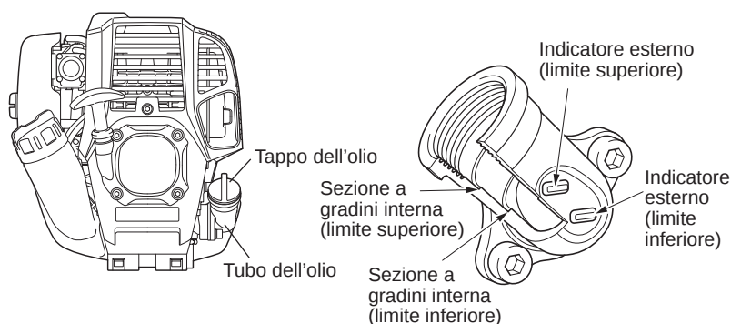
Fig. 2 Tubo dell'olio
