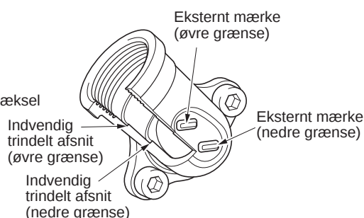
Fig. 2 Olierør
