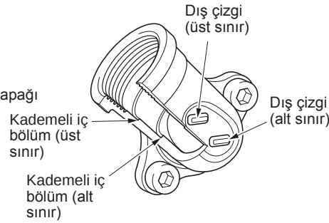
Şekil 2 Yağ borusu
