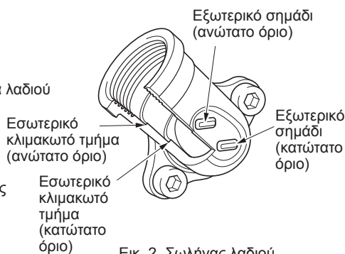
Εικ. 2 Σωλήνας λαδιού
