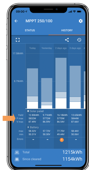
VictronConnect-App mit Historie Pmax-Wert.
