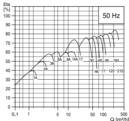
Obr. 1 Stupeň účinnosti čerpadla/motoru v závislosti na průtoku
