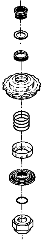
Obr. 12 Ucpávka hřídele, MS 4000
