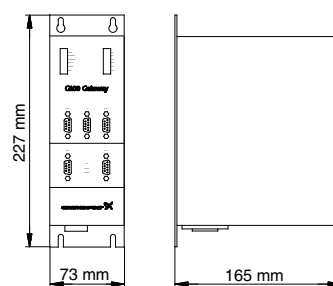
Obr. 24 Rozměrový náčrtek
