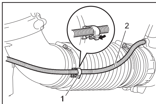
► 1. Držák lanka 2. Ovládací lanko
