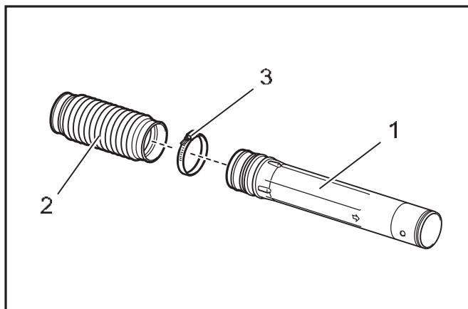
► 1. Otočná trubka 2. Ohebná trubice 3. Hadicová páska
