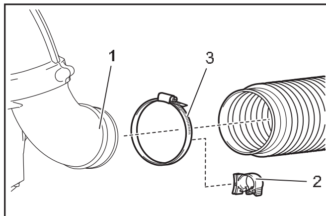
► 1. Koleno 2. Držák lanka 3. Hadicová páska
