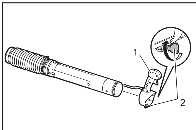
► 1. Ovládací páka 2. Šroub spojky
