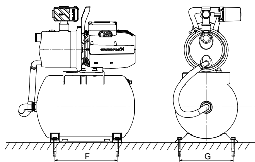
Obr. Základ zvyšovacího čerpadla JP PT-H
