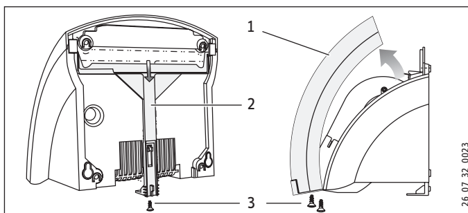
1 Capot de boîtier 2 Verrou 3 Vis
