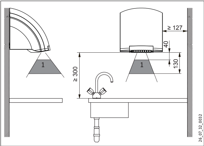
1 Az infravörös közeltítésérzékelő érzékenységi területe
