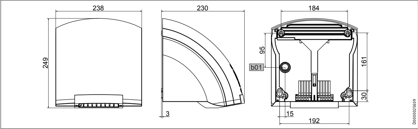
b01 Doorvoer elektrische kabels (Achteraanzicht van het toestel)
