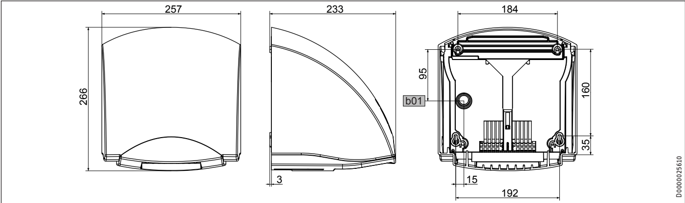
b01 Przepust na przewody elektr. (widok urządzenia z tyłu)
