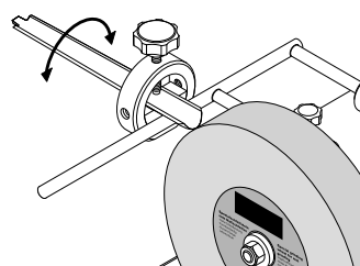
Dispositif pour tuyaux et fer creux (avec 100) 55, n° de commande 8949 0706
