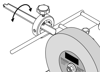
Prípravok pre rúrky a duté profily (100) 55, kat. č. 8949 0706
