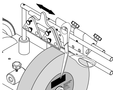
Przyrząd do nożyc (z 100) 160, nr zamów. 8949 0710 Nożyczki do papieru, materiału czy też nożyce do żywopłotu - teraz naostrzycie Państwo wszystkie!
