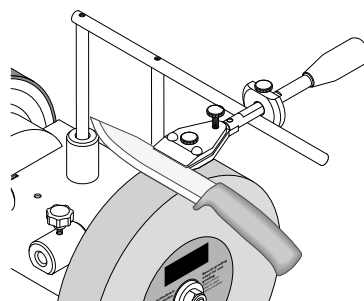
Dispositif pour petits couteaux 60, n° de commande 8949 0708
