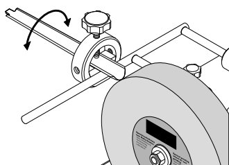
Jig til flad- og skråmejsler og billedskærerjern og – mejsler, bestillingsnr. 8949 0706 , Jig 55
