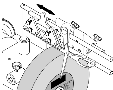
Jig til sakse, bestillingsnr. 8949 0710 , Jig 160
