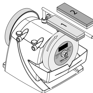
Prépare meule, n° de commande 8949 0707
