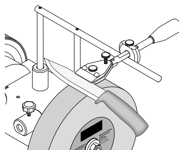
Prípravok pre malé nože 60, kat. č. 8949 0708
