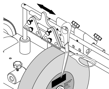
Dispositif pour ciseaux et cisailles (avec 100) 160, n° de commande 8949 0710
