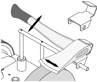
Werkstukhouder 40, voor bijlen, bestel-nr. 8949 0712 Moeiteloos brandhout hakken, en zonder grote machines
