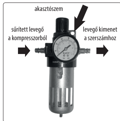
9. ábra. Nyomásszabályozó manométerrel és szűrővel, Extol® 8865104
