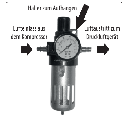
Abb. 9 - Beschreibung vom Druckregler mit Manometer und Filter Extol® 8865104
