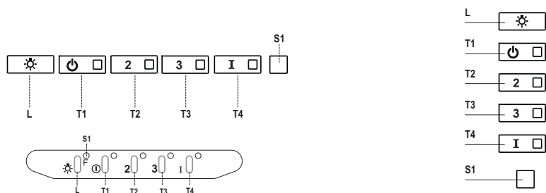
Ovládací panel
