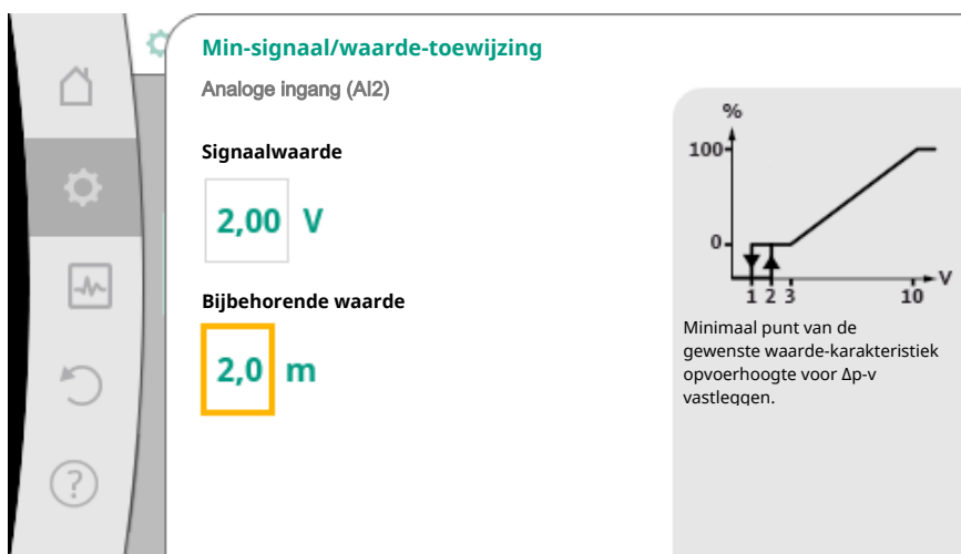
Fig. 75: Min-signaal/waarde-toewijzing
