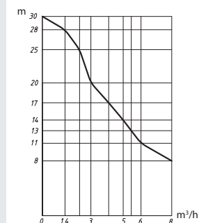
Graf 1; průtokový graf čerpadla 414502
