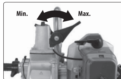
Abb. 5, Position vom Hebel der Durchflussregelung für Min. und Max.
