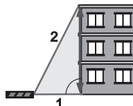
Obr. 1, funkcia jednoduchého pytagoriánu
