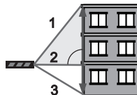
Obr. 2, funkce dvojitého Pythagoriánu
