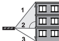
Obr. 2, funkcia dvojitého pytagoriánu
