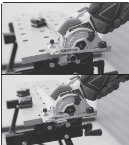
Abb. 21, Sägen eines Aluminium-Rohres und einer Eckleiste
