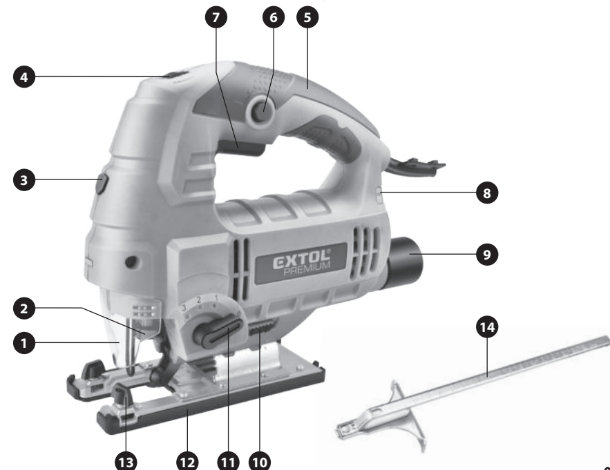
Obr. 5, Pozícia – popis
