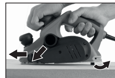
Obr. 5 C, sklopenie trňa na plochu
