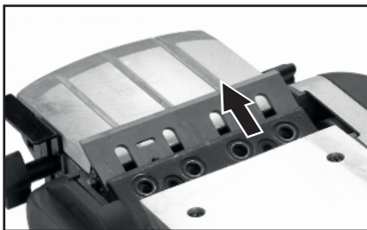
Obr. 9, vyňatie noža u modelu hoblíka EP 1300
