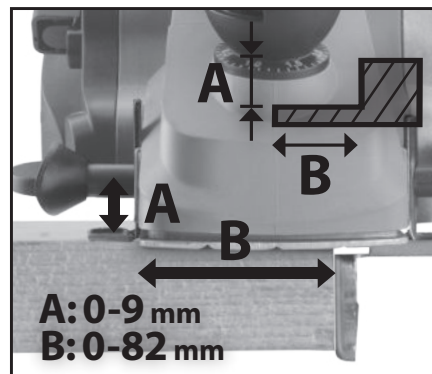
Obr. 7, profil polodrážky; nastavenie rozmerov polodrážky na hoblíku
