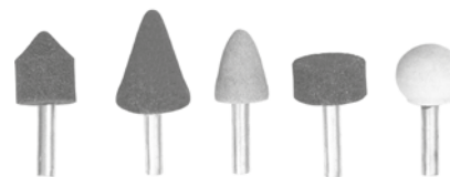
1. ábra - Az Extol Craft 1820 csiszolószerszám készlet
