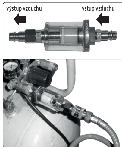
Obr. 6, připojení filtru (odlučovače) Extol® Craft 8865101
