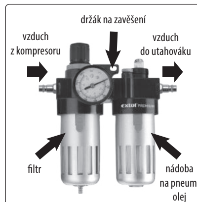
Obr. 8, popis úpravné jednotky Extol® 8865105
