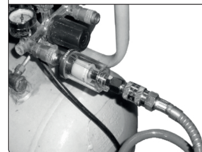
6. ábra. Extol® Craft 8865101 szűrő (leválasztó) bekötése
