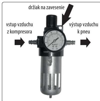
Obr. 7, popis regulátoru tlaku s manometrom a filtrom Extol® 8865104
