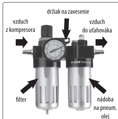
Obr. 8, popis jednotky na úpravu Extol® 8865105
