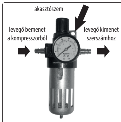
7. ábra. Nyomásszabályozó manométerrel és szűrővel, Extol® 8865104
