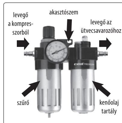
8. ábra. Extol® 8865105 levegő előkészítő egység
