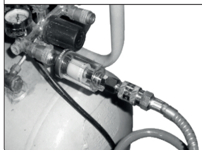
Abb. 6, Anschluss vom Filter (Abscheider) Extol® Craft 8865101
