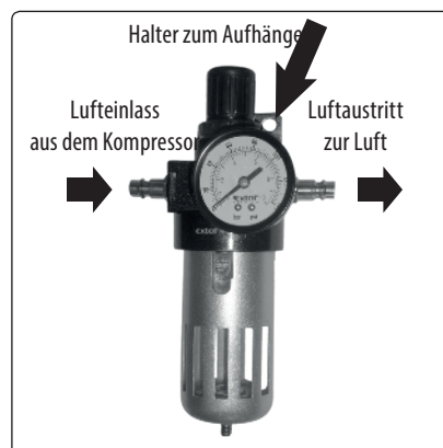
Abb. 7 - Beschreibung vom Druckregler mit Manometer und Filter Extol® 8865104
