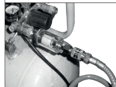
Obr. 6, pripojenie filtra (odlúčovača) Extol® Craft 8865101
