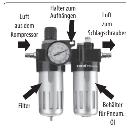
Abb. 8, Beschreibung der Aufbereitungsanlage Extol® 8865105
