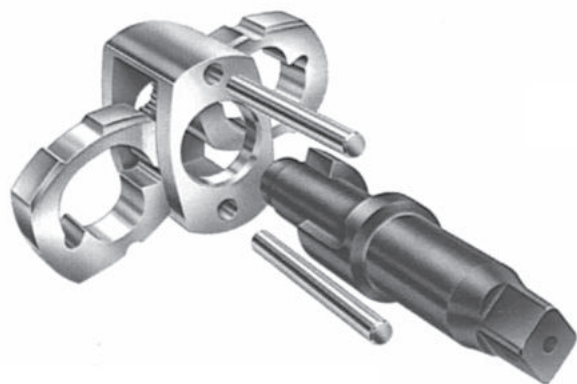
1. ábra. A „Twin hammer” rendszer
