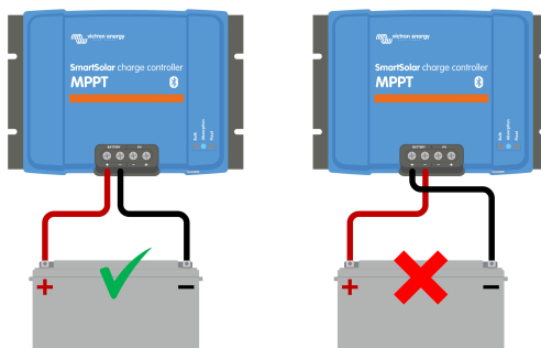
Exemples de polarité correcte et incorrecte (inversée) de la batterie.
