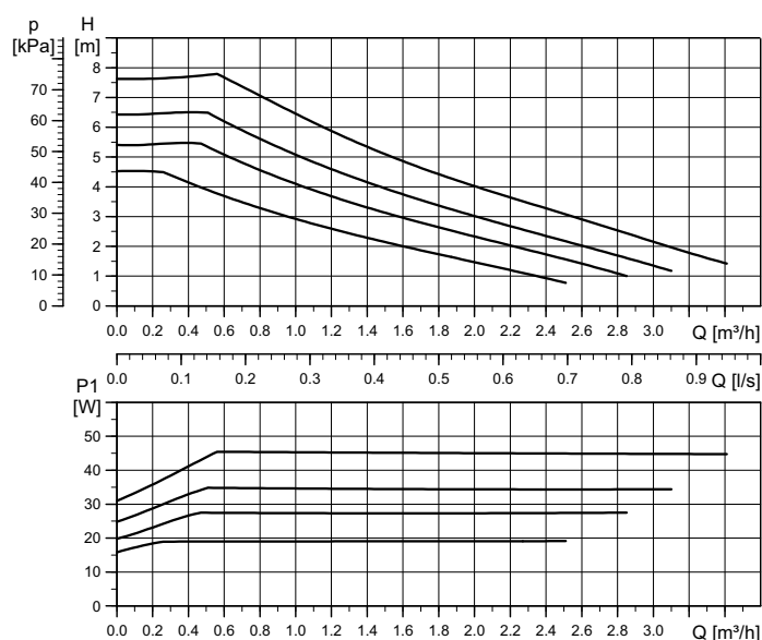
Obr. 51 Výkonová křivka
