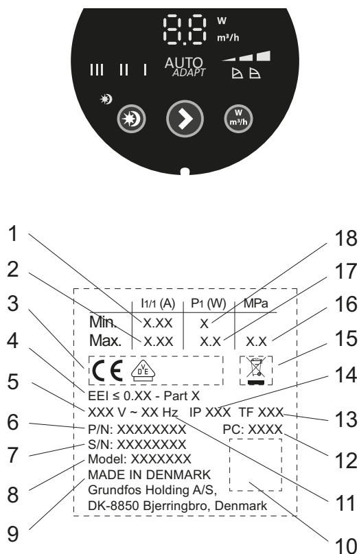
Obr. 18 Typový štítek
