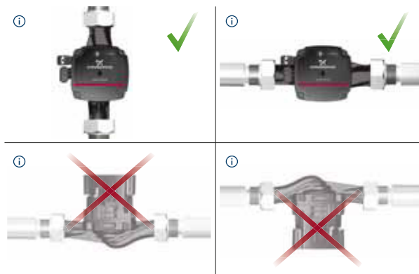
Obr. 7 Umístění řídicí jednotky ALPHA SOLAR
