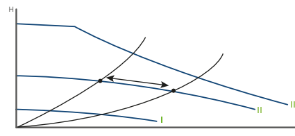
Obr. 28 Nastavení tří konstantní křivky/konstantní otáčky
