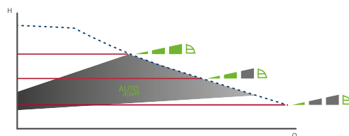
Obr. 23 Volba nastavení čerpadla pro určitý typ soustavy
