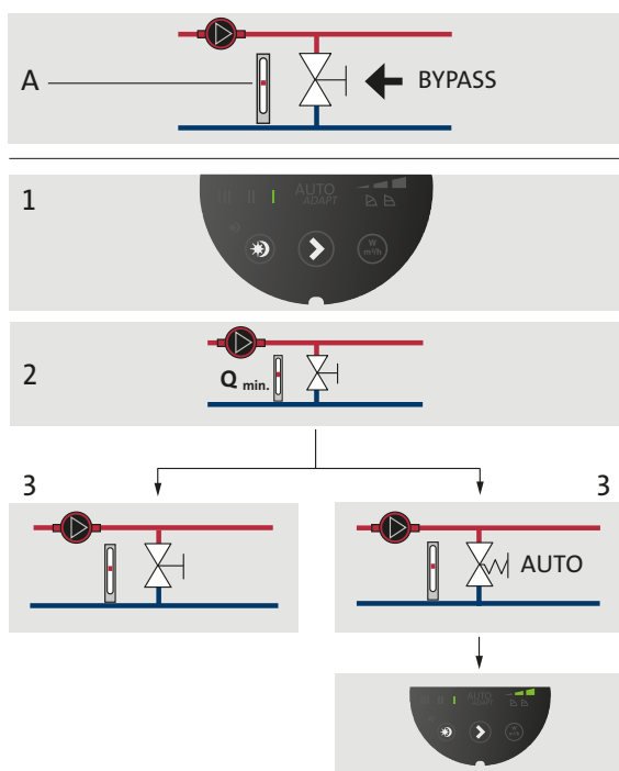
Obr. 30 Soustavy s obtokovým ventilem
