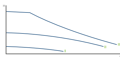
Obr. 27 Volba nastavení čerpadla pro určitý typ soustavy
