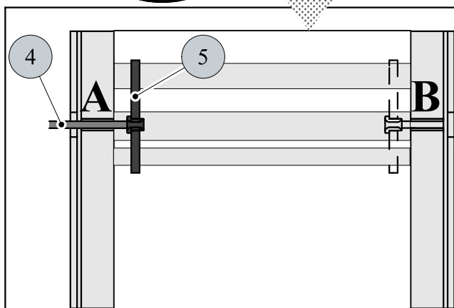
Informativní náhled do prostoru kamen při čištění výměníku
