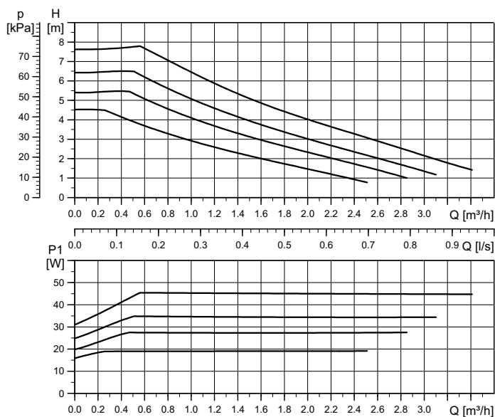
51. ábra Jelleggörbe
