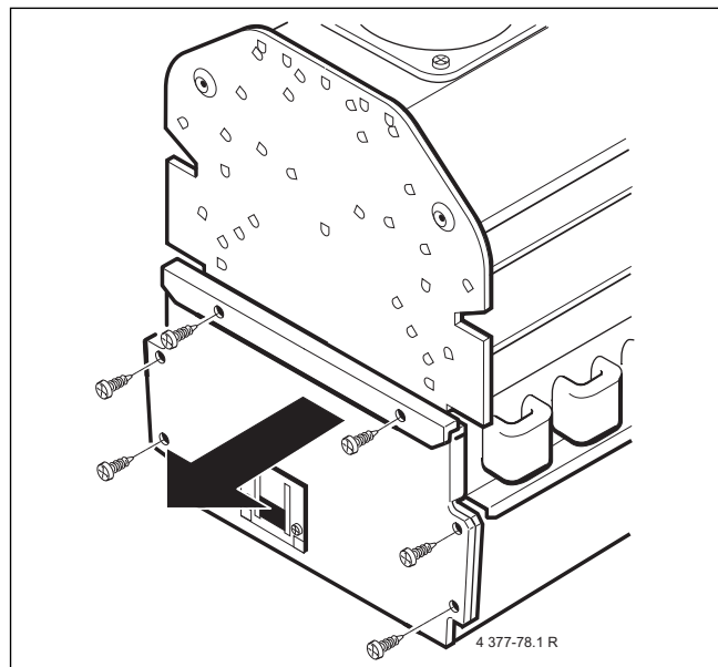
Obr. 53 ZSR 10-7 KE..
