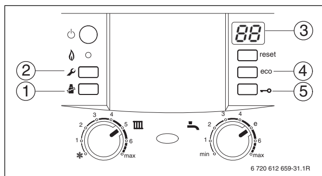
Obr. 40 Přehled ovládacích prvků
