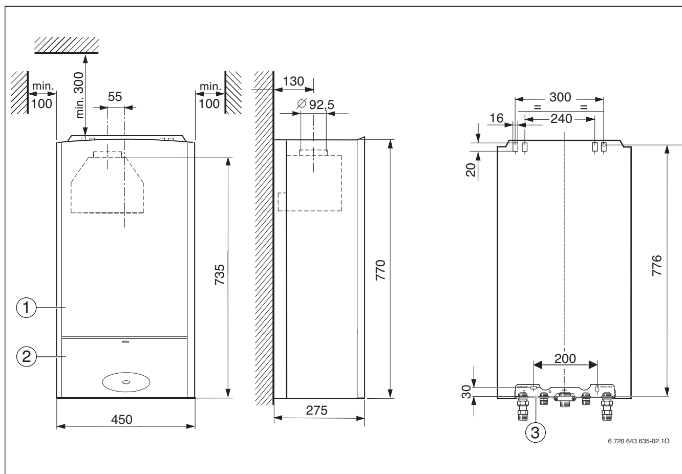
Obr. 3 ZSR 10-7 KE
