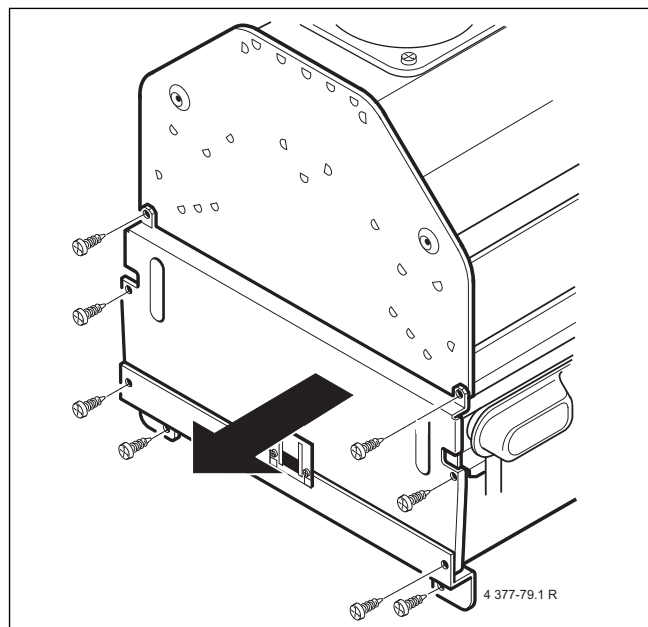
Obr. 54 ZWR/ZSR 18/24...-7 KE..
