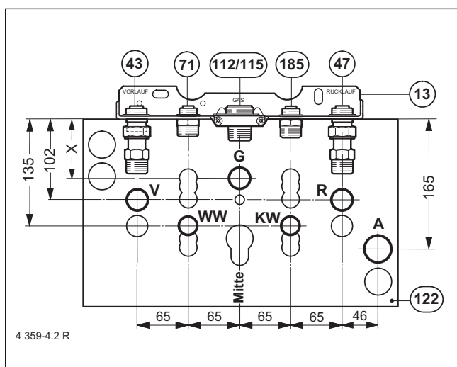
Obr. 11 Připojovací rozměry s montáží pod omítku
