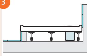
Podezděním a obložením
