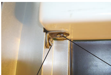
Použít šrouby 4,2x12 Svislé profily spojit se střešou use screws 4,2x12, link the vertical profiles with top panel
