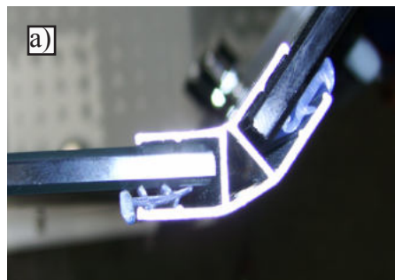
Utěsňit těsněním seal...
