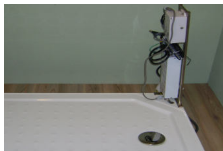
Instalovat generátor install the generator
