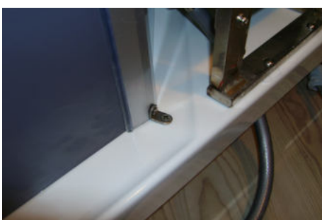
Použít šrouby 4,2x12 Svislé profily spojit s vaničkou use screws 4,2x12, link the vertical profiles with shower tray
