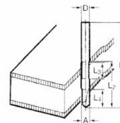
Dvojitá lícovací frézka
