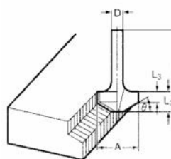
Frézka na úhlové hrany
