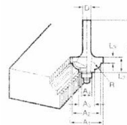
Profilové frézka s náběhovým kuličkovým ložiskem
