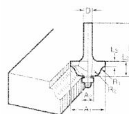
Profilové frézka s náběhovým kuličkovým ložiskem
