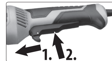
Obr. 6, Odjištění (krok 1.); zapnutí (krok 2.)
