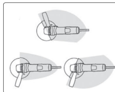
Obr. 3, řezné zóny kotouče a natočení ochranného krytu kotouče ve vztahu k držení a postoji obsluhy
