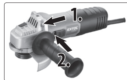
Obr. 5, zapnutí (krok 1.); aretace (krok 2.)
