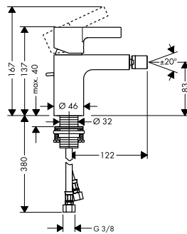
Metris S 31261000
