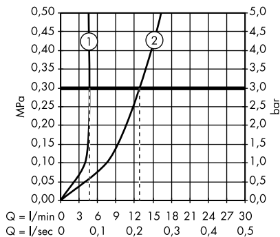
Metris S 31060000 / 31066000 / 31068000
