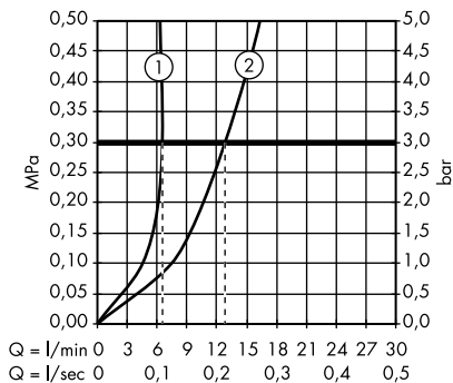
Metris S 31261000
