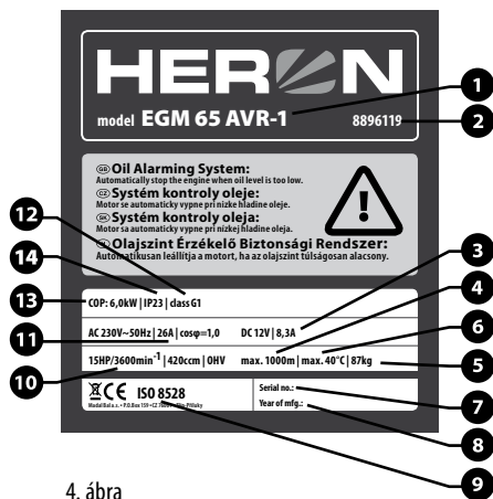
4. ábra: adattábla (1. ábra, 3. pozíció)
