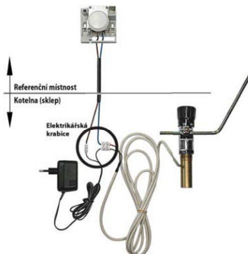
Obr. 4 – termostát spíná 12 V, kontakty musí být dimenzovány na 1 A (zapojení a názorný obrázek)
