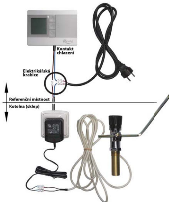
Obr. 5 – termostát spíná 230 V, kontakty musí být dimenzovány na 230 V / 200 mA (zapojení a názorný obrázek)
