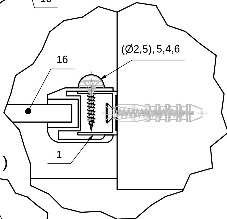
G ( 1 : 1 )
