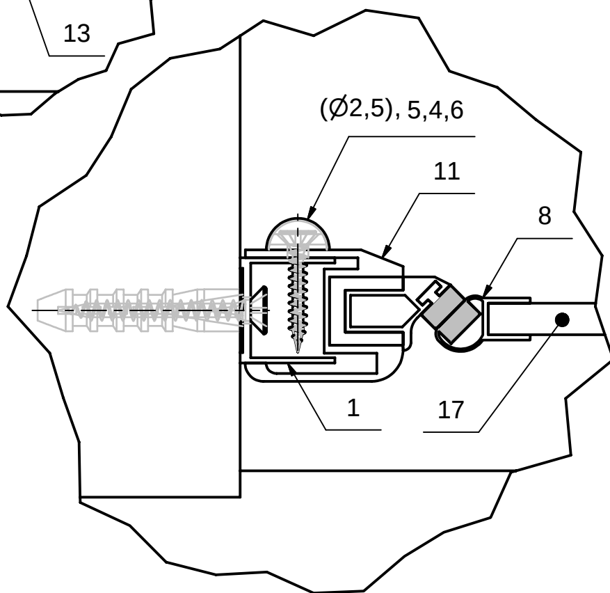
J ( 1 : 1 )
