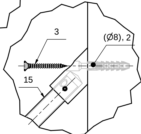
E ( 0,60 : 1 )
