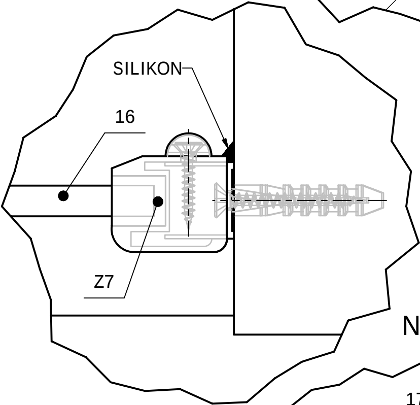
M ( 1 : 1 )
