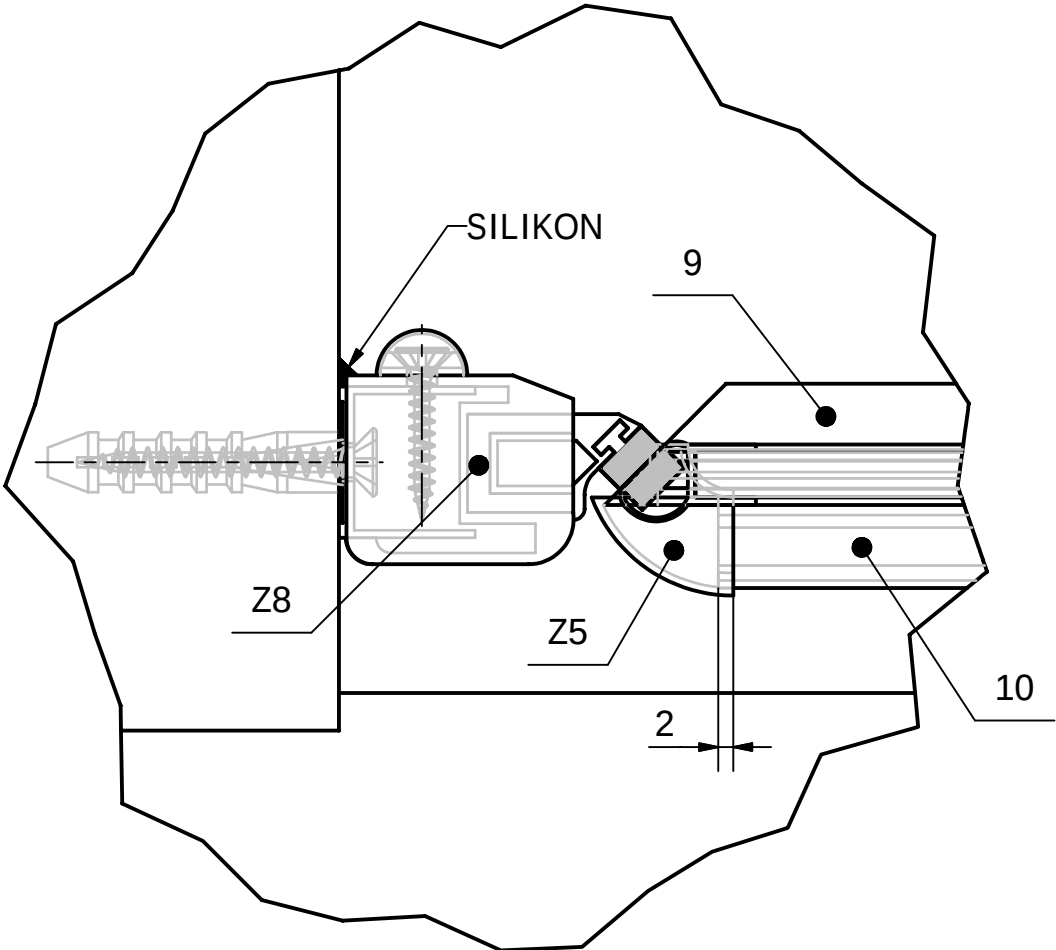
P ( 1 : 1 )
