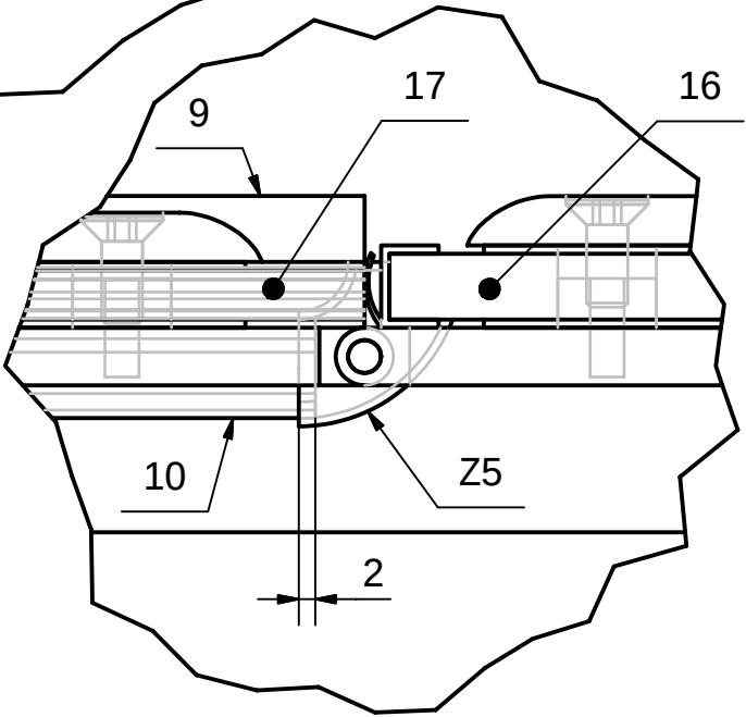
N ( 1 : 1 )
