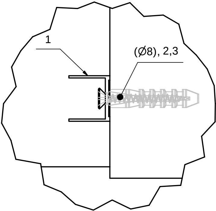
B ( 1 : 1 )
