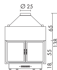
IDRO 100 Dvoukřídlá zasouvací dvířka
