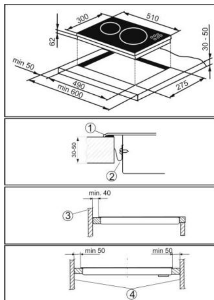
1. Uszczelka, 2. Docisk, 3. Ściana tylna, 4. Ściany boczne
