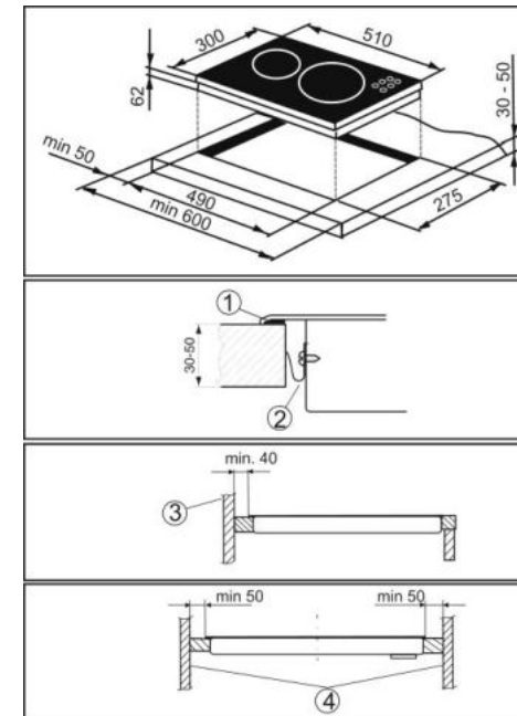
1.Tömítés, 2.Szorító, 3. Hátsó fal, 4. Oldalfalak
