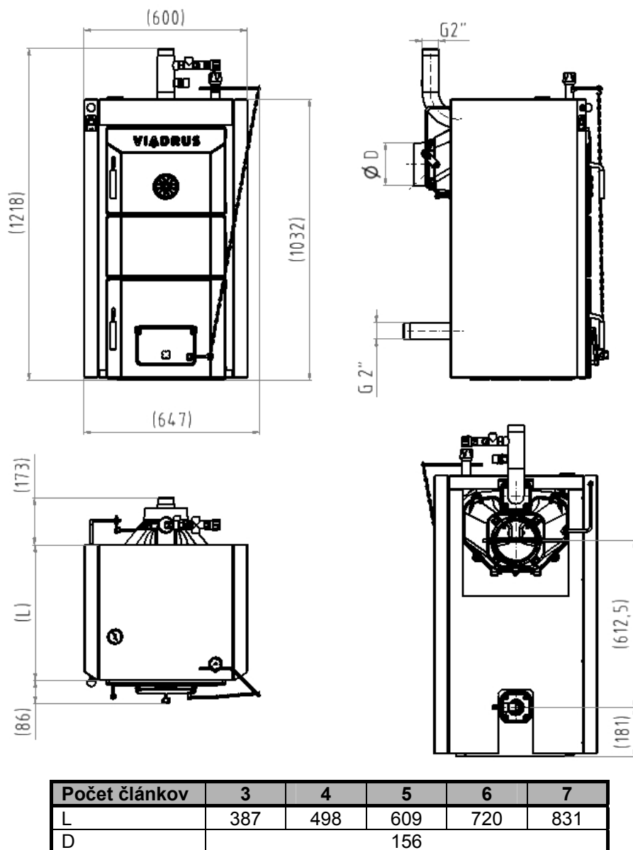
Obr. č. 10a) Pripájacie rozmery kotla VIADRUS HERCULES U 26 3 – 7 čl.
