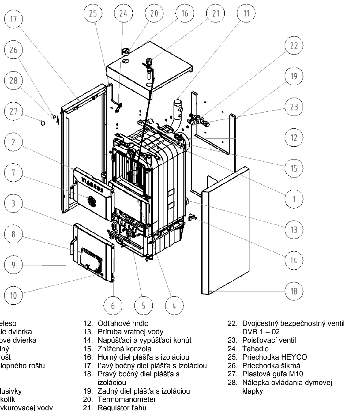
Obr. č. 3a) Zostava kotla VIADRUS HERCULES U 26 3 – 7 čl.
