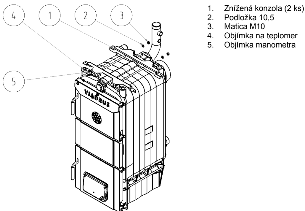
Obr. č. 12 Montáž konzol plášťa
