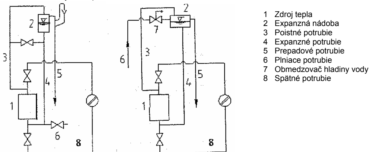
Obr. č. 7 Príklady zapojenia otvorených expanzných nádob
