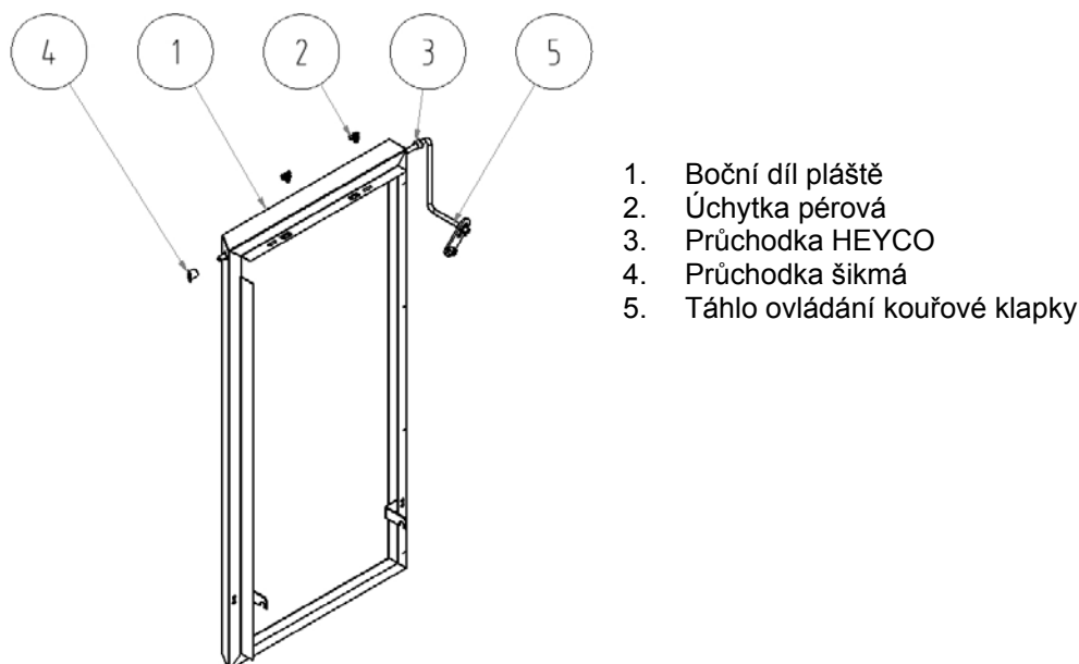
Obr. č. 14 Levý boční díl pláště
