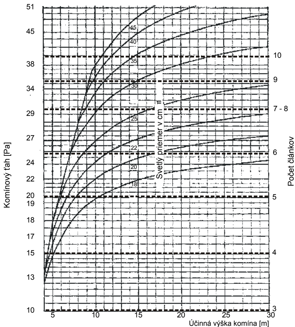
Obr. č. 2 Stanovení priemeru komína
