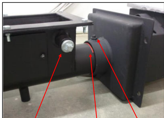
Jímka pro voskovou patronu zálevového systému
