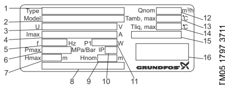
Obr. 1 Typový štítok
