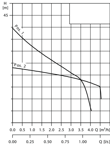
Fig. 3 Curva QH y posiciones de la válvula eyectora
