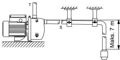
Joonis 2 Torude ühendamine
