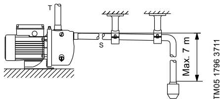
Slika 2 Povezivanje cevi
