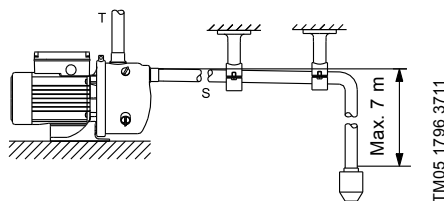
Fig. 2 Attacco tubazione
