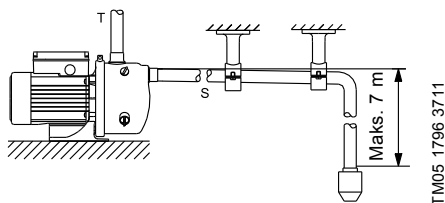
Slika 2 Cevni priključki
