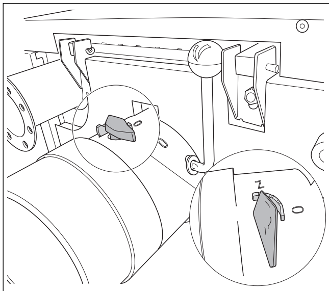
Obr. 6 Nastavení spalínové klapky
