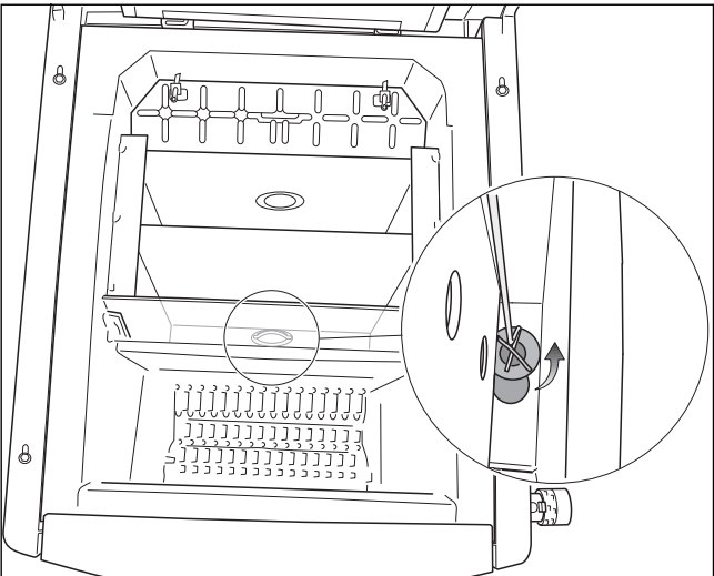
Obr. 18 Odstranění čisticího víka
